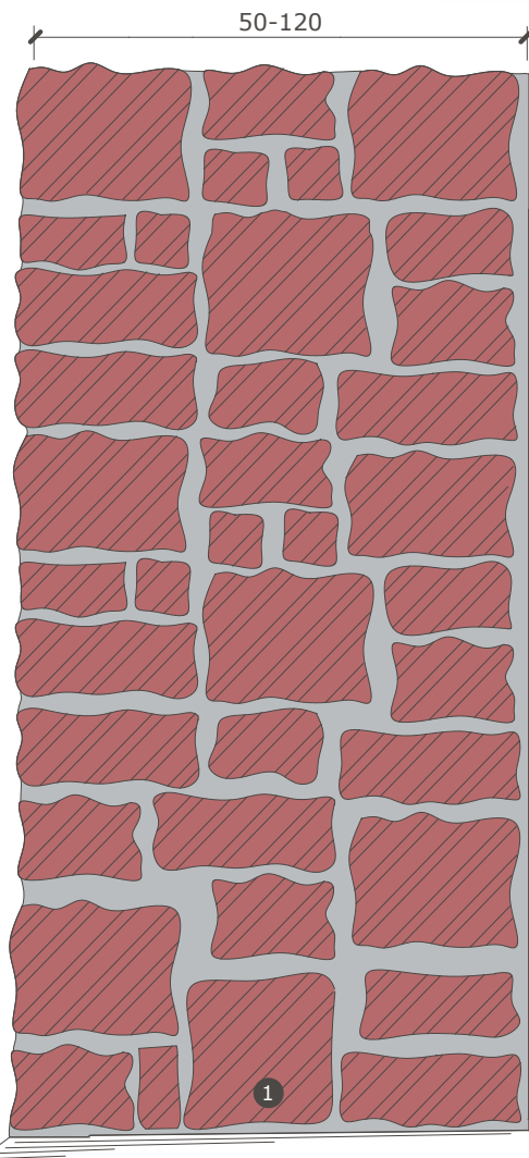
1 Natursteinmauerwerk, massiv
